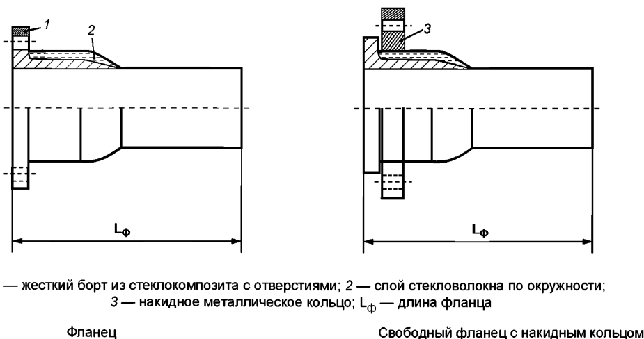
Рисунок 8 — Фланцы
