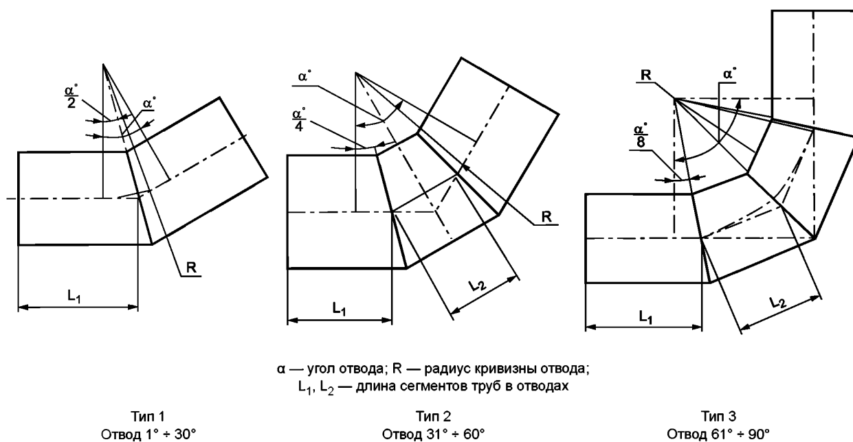
Рисунок 5 — Отводы
