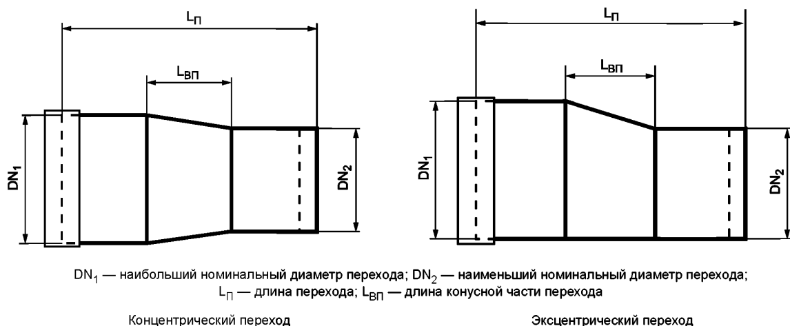
Рисунок 6 — Переходы
