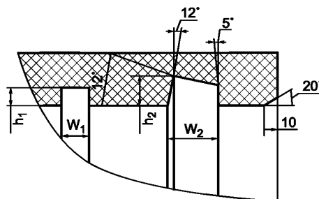
h_1 — глубина канавки под центральный ограничитель; h_2 — глубина канавки под уплотнительные кольца; W_1 — ширина канавки под центральный ограничитель; W_2 — ширина канавки под уплотнительные кольца
